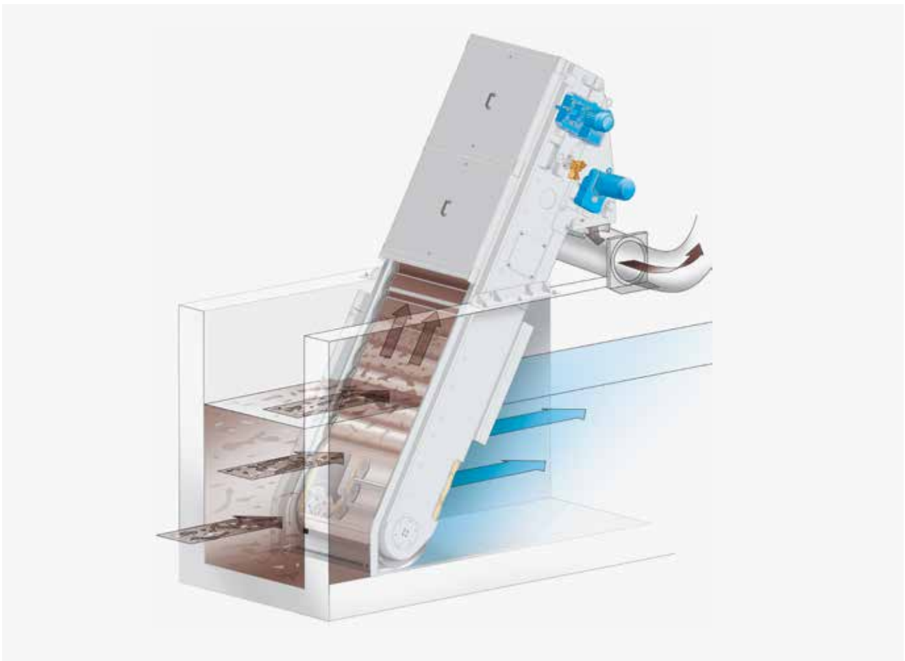
Schematische Darstellung des HUBER Lochblech-Umlaufrechen EscaMax®.
