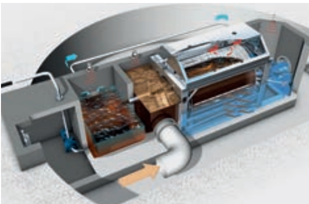
Darstellung CarbonWin®-Verfahren: Das bessere Vorklärbecken für optimale Reduktionsraten (siehe Einzelprospekt).
