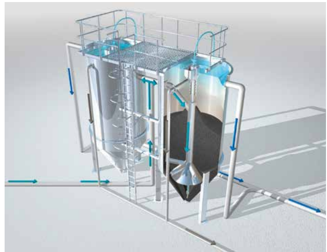
HUBER Aktivkohlefilter CONTIFLOW® GAK (Behälterversion).
