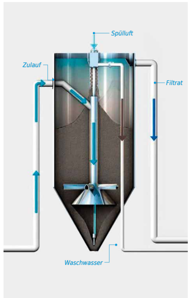
Prinzip HUBER Aktivkohlefilter CONTIFLOW® GAK.
