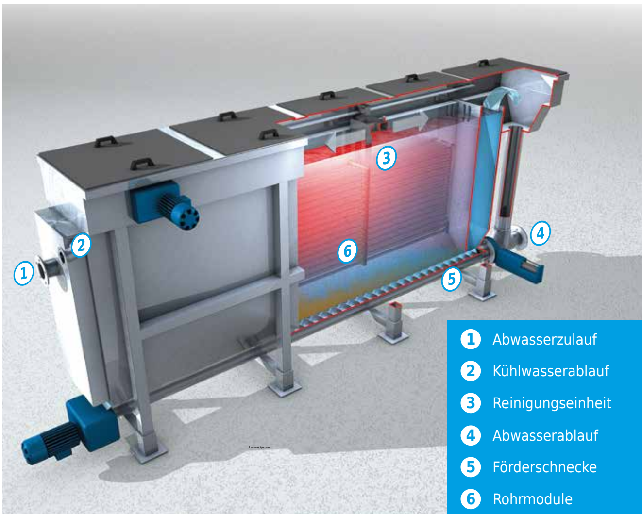
Schematische Darstellung des HUBER Abwasserwärmetauschers RoWin.
